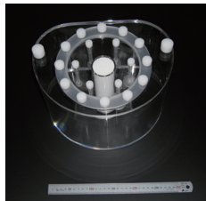
PET・MRI・CT 検査の評価 ファントム
