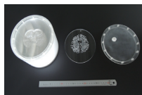
3D 脳ファントム (人の頭をイメージして作成、灰白質・白質・ 脳質の構造)
